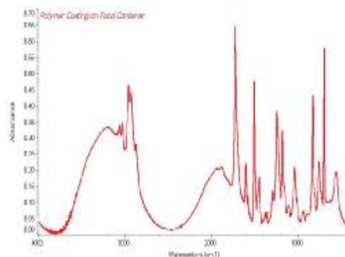
30度镜反射附件测量食品包装材料上聚合物涂层红外光谱图
