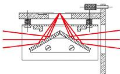
30 度镜反射附件光路示意图
